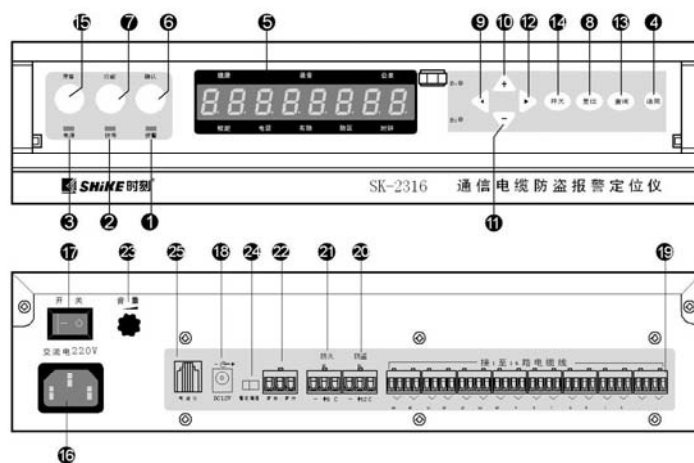
SK-2316面板 接线板
