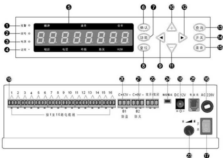
SK-2316B面板 接线板
